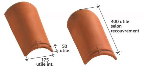
Faitière / Arêtier pureau variable à emboîtement (2,5 au ml) (3) Réf. 708 - clips de faitière pureau variable Réf. CR101
