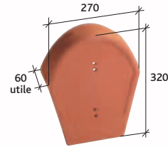
Fronton 90° grand modèle pour faitières pureau variable à emboitement (grande ouverture) et rabat (3) Réf. 814
