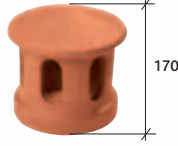
Lanterne ø 100 utile (section d'aération : 130 cm 2 ) Réf. 1005
