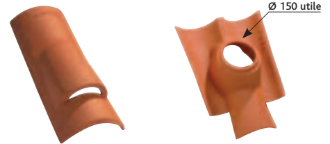
Tuile chatière Canal (1) (section sans grille = 21 cm 2 ) Réf. 403.21
